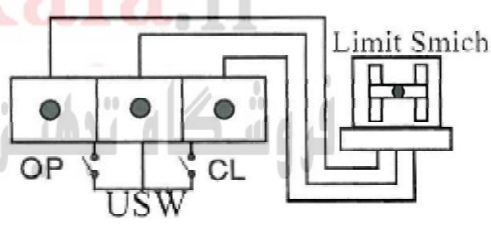
۶- لیمیت سوئیچ
