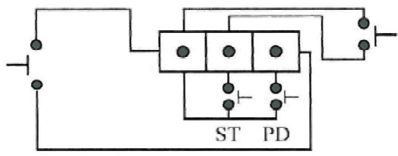
۱- استارت دولنگه
