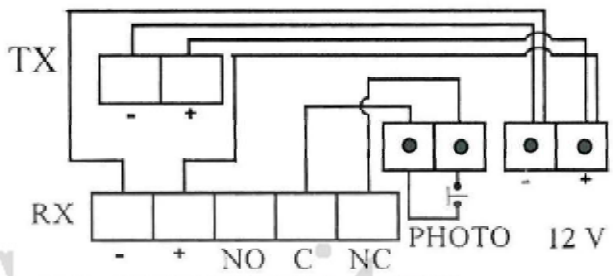
۴- چشمی
