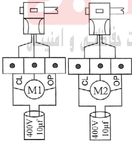
۷- موتور
